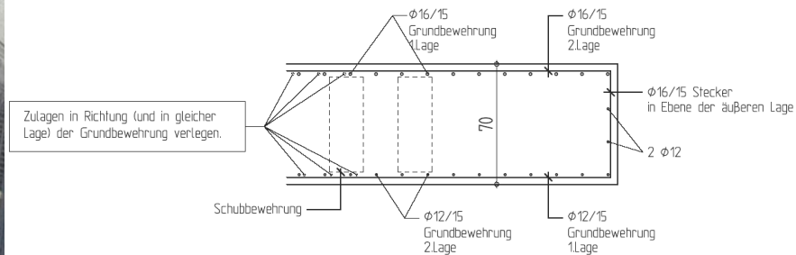
Schnitt 1 M=1:25
