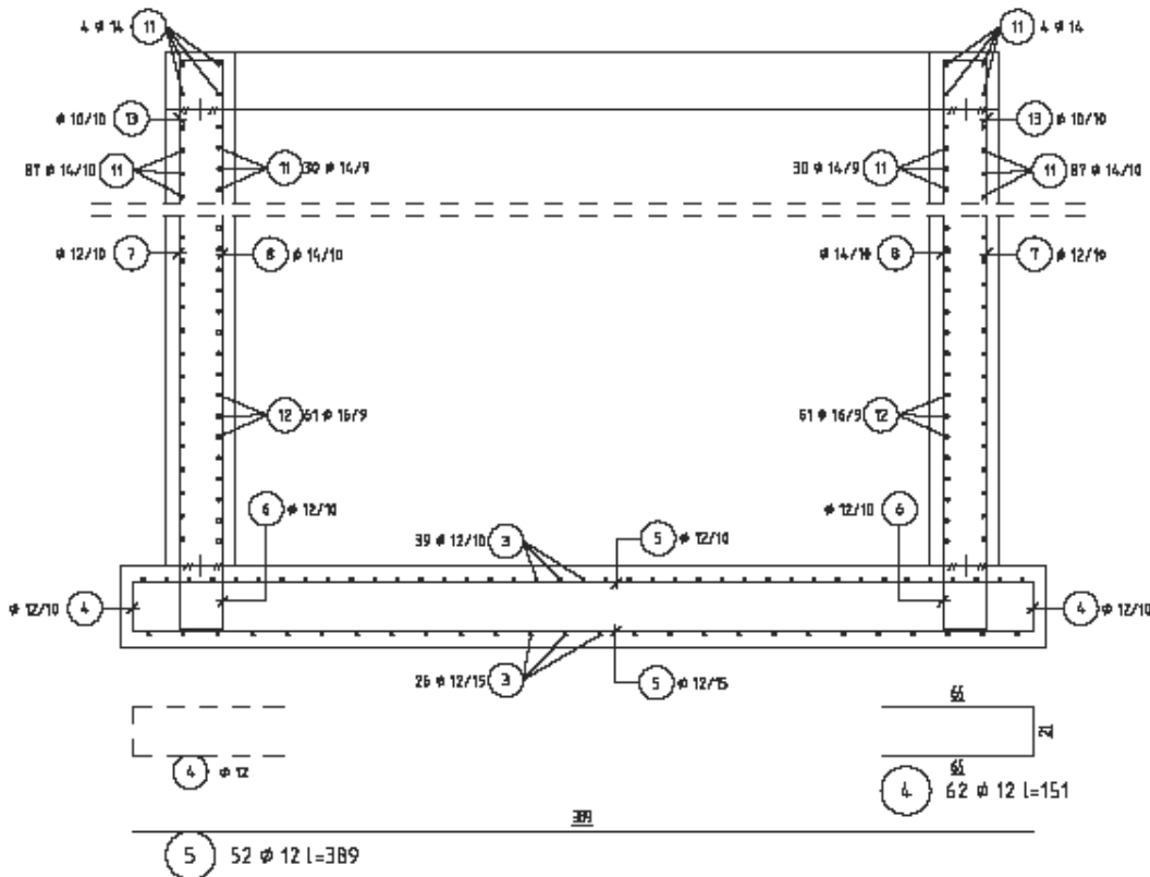
Schnitt 2 M=1:25
