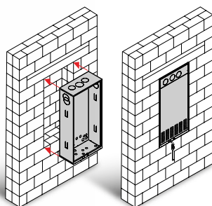
Montaggio dell'unità da incasso di KON m INC
