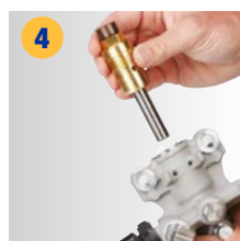
4 Neue Patrone installieren und Pumpe einsetzen
