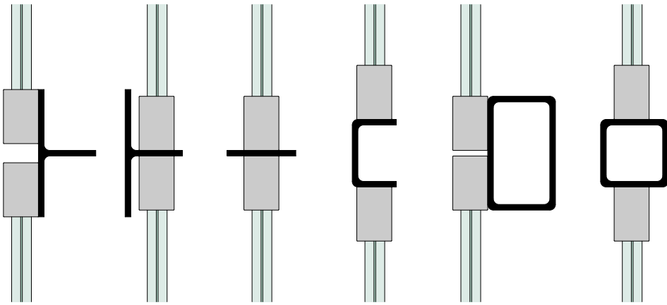
Stahlprofile z. B. Geländerpfosten
