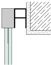
Rollladenschiene auf Mauerwerk
