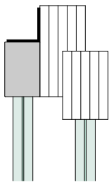
Seitlich mit Winkel (Holzprofil)
