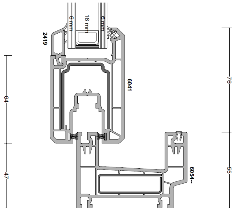
TELAIO 6054 + ANTA 6041
