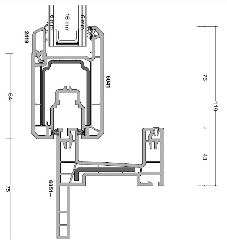
TELAIO 6051 + ANTA 6041
