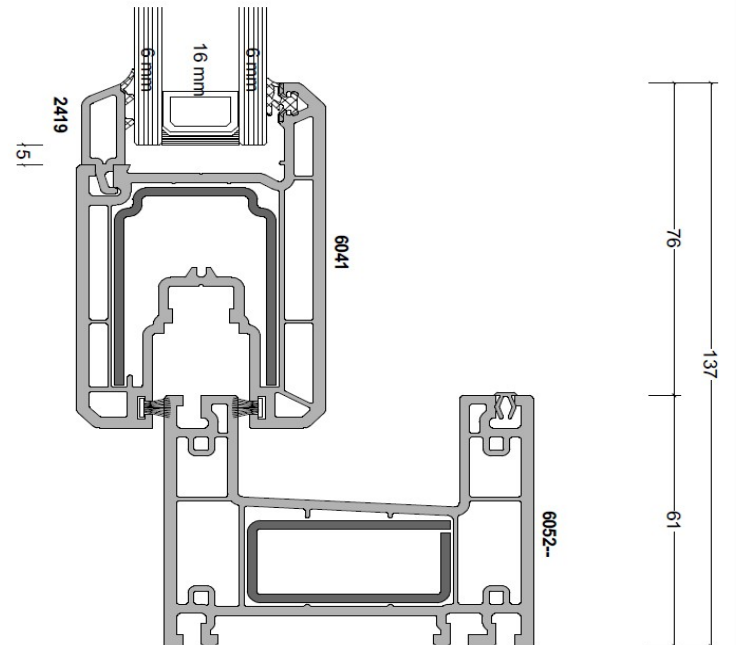
TELAIO 6052 + ANTA 6041
