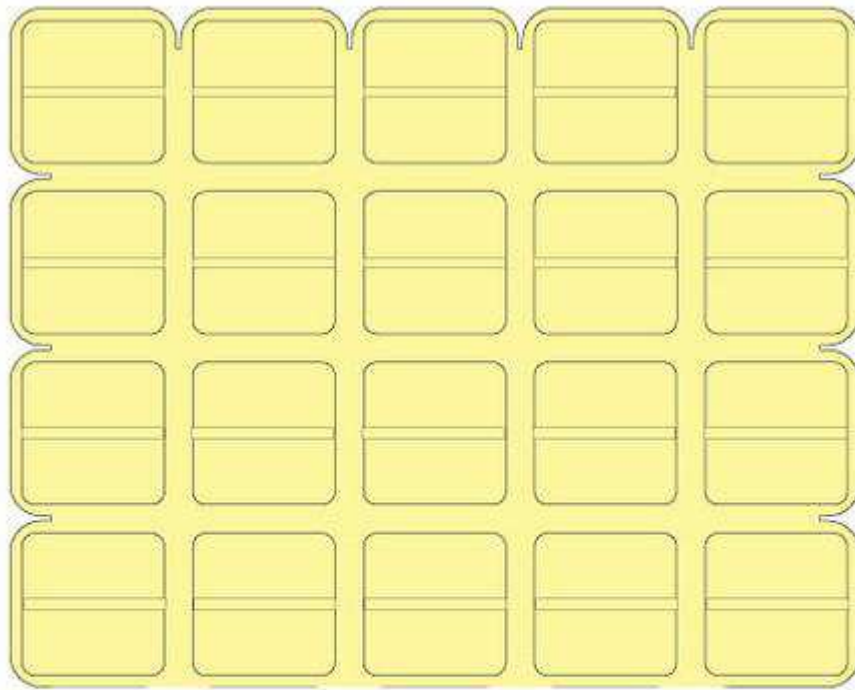
Karte 4 x 5 Chips Chip = 23 x 23 mm Bruchlinie doppelseitig
