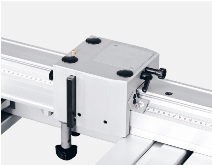
2-Punkt-Längenanschlag | T60A40
