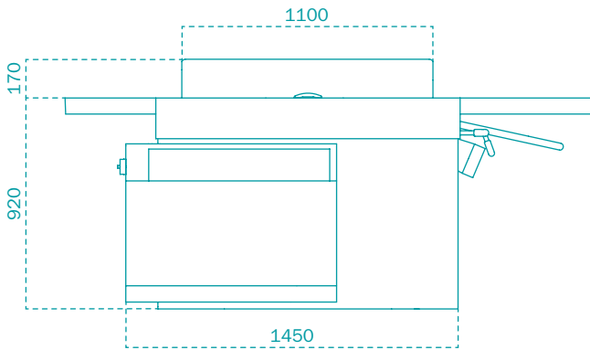
TP300 | Seitenansicht
