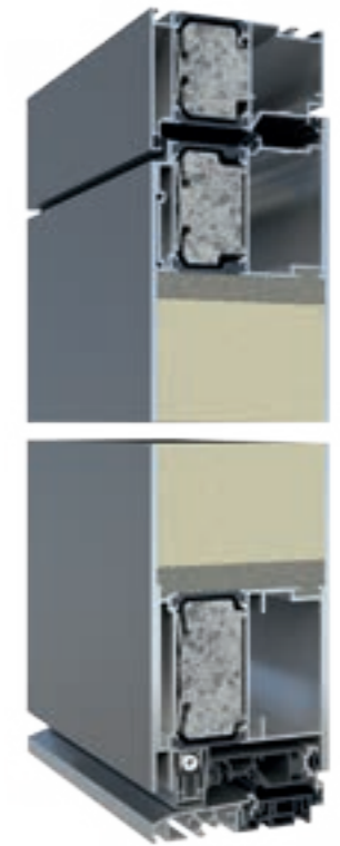
KOtherm 96 in Ausführung beidseitig flügelüberdeckend
