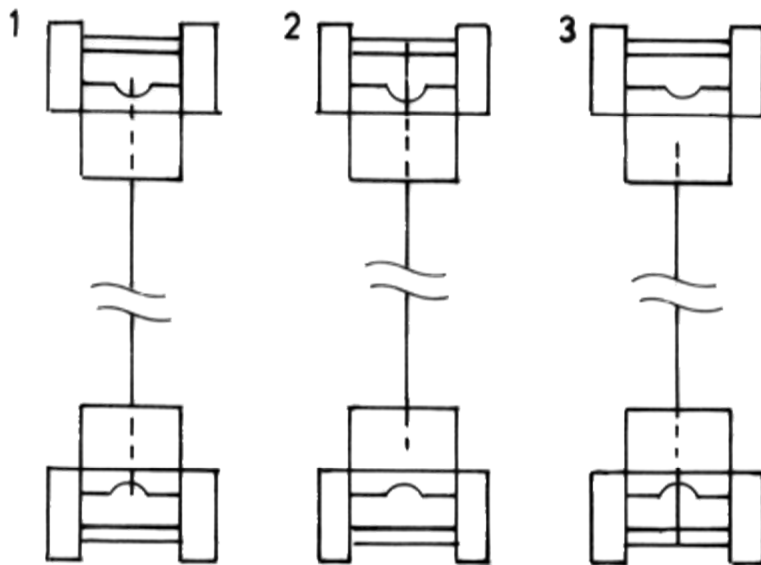
Abb. 7. Dreimaliger Einsatz eines Blattes durch Umspannen.
