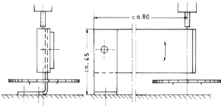
Abb. 4: Plexiglas-Schutzschild zum Sägen von Kleinteilen.
