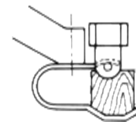
Abb. 6. Formklemmstück.
