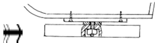
Abb. 1: Die Drehaufnahme
