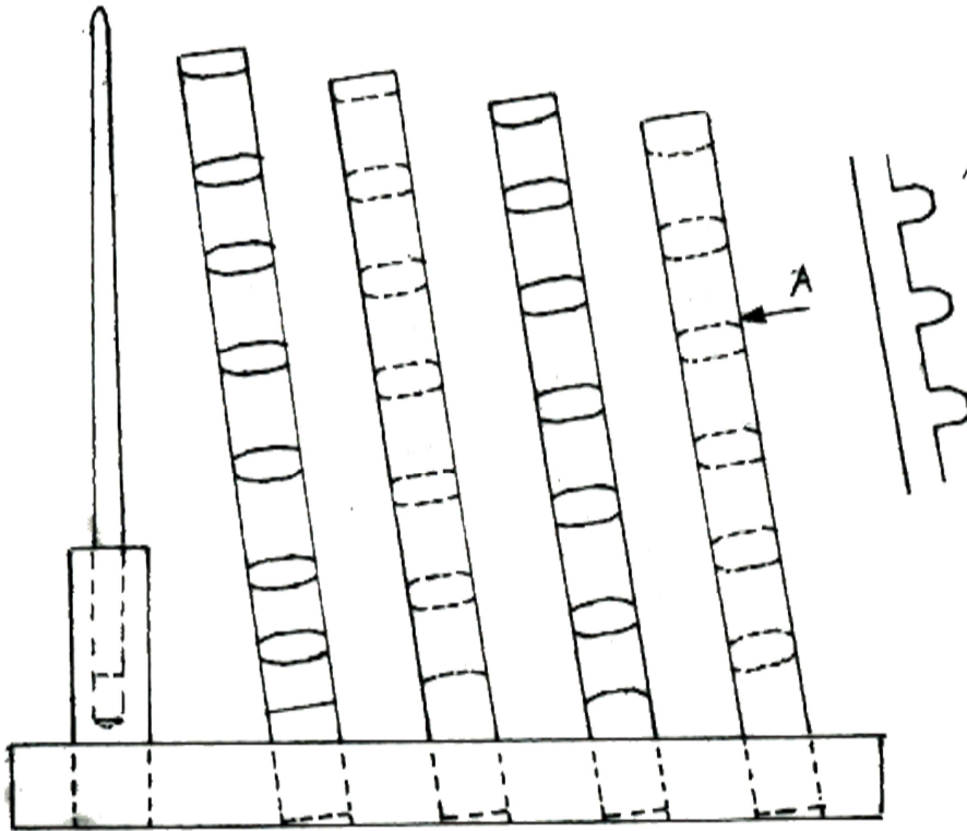
Abb. 10: Fahnen-Biegevorrichtung
