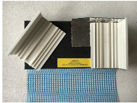
V-5: emv-PVC Slider U passend für den Einsatz bei verputzten Leibungen ohne Leibungsplatten (Slider U)
