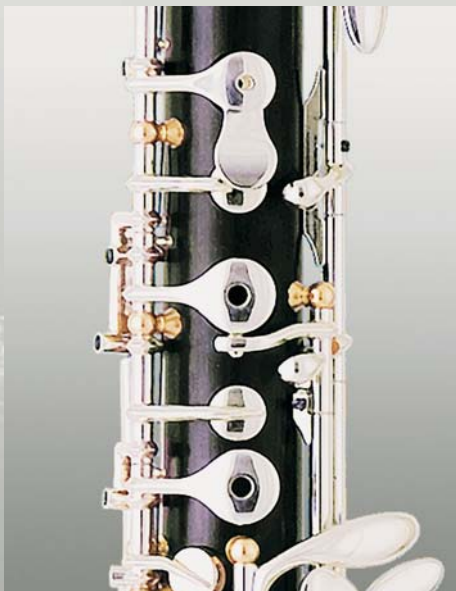
einteilige Halblockklappe
