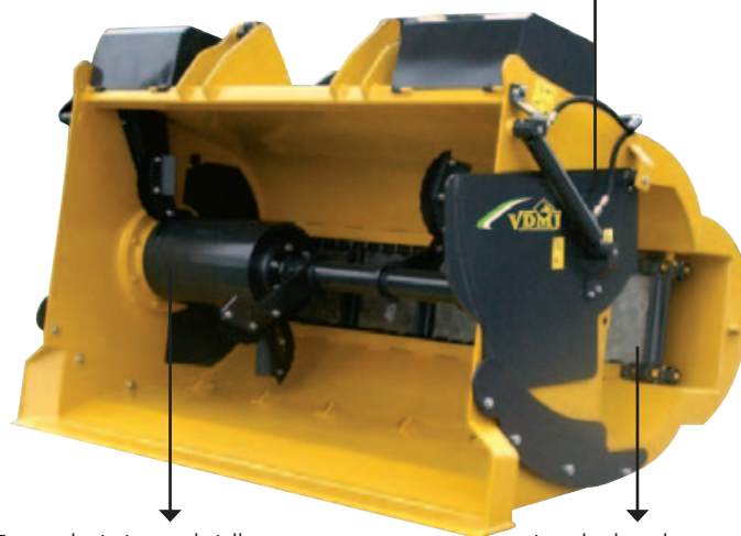
Zware planitaire tandwielkast als aandrijving op menger. D'entraînement avec un batteur forte réduction planétaire.
