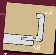
Zarge RR als Schnittzeichnung
