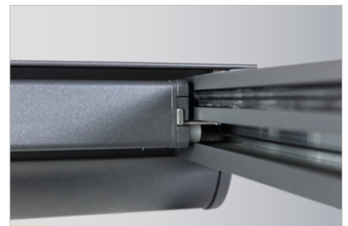
Führungsschiene mit Fallstange
