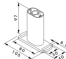
W500 Standard-Montagekonsole
