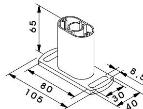
W450 Standard-Montagekonsole
