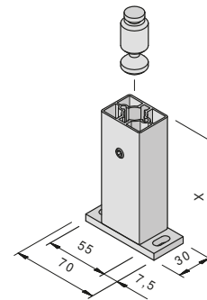
W350 Führungsschienenhalter X = 90 (Standard), 150, 200, 300 mm (nur ohne Zip)
