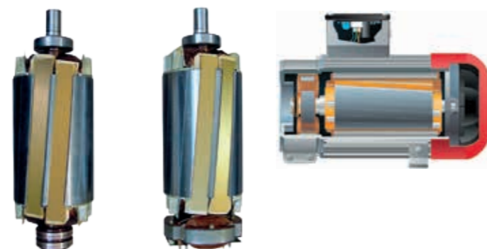
Rotorkopf mit verschleißanfälligem Kohle-Bürstenbetrieb
