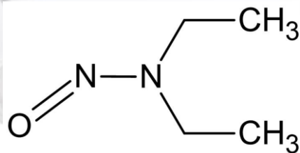
N-Nitrosodiethylamine
