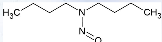
N-Nitrosodibutylamine
