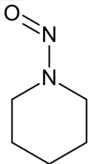
1-Nitrosopiperidine
