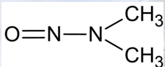
N-Nitrosodimethylamine
