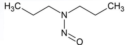
N-Nitrosodi-n-propylamine
