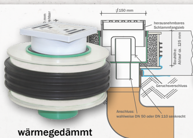
mit Folienflansch öl- und bitumenbeständig
