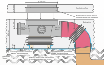
Kellerablauf mit Kunststoffrost
