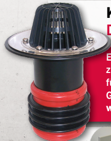
KRASO® Bodenablauf Aufsatzrahmen mit Bauzeitschutzdeckel für Industrieböden die mit einem Flügelglätter behandelt werden
