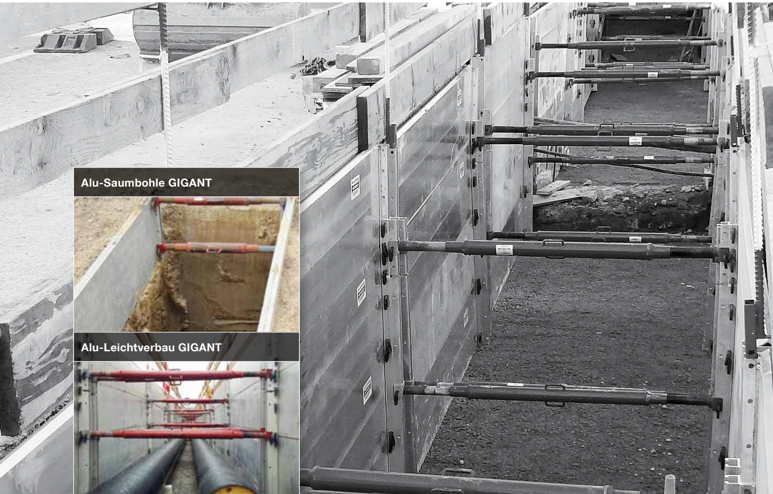
Alu-Kammerplattenverbau GIGANT
