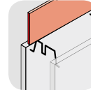
Wandkopfabdichtung Fradiflex® ohne Befestigungswinkel mit Fixierbügel
