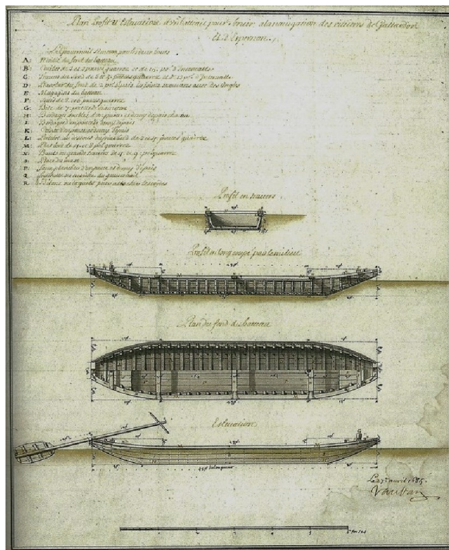
Vauban – Projet de bateau pour servir à la navigation des rivières de Gallardon et d'Epernon (27 avril 1685)
