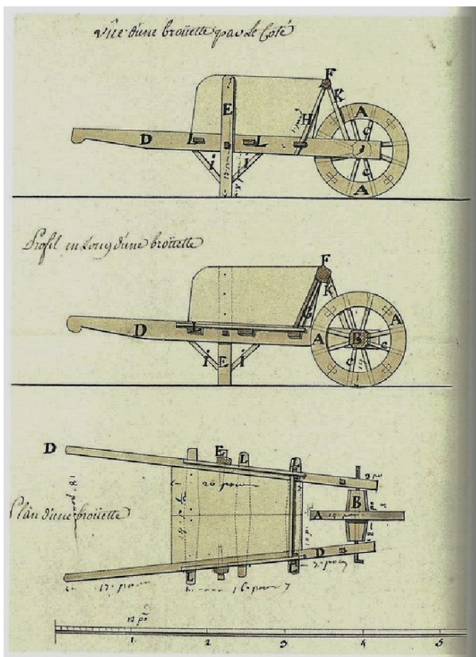
Vauban – Modèle de brouette utilisée pour le terrassement des chantiers du Canal de l'Eure
