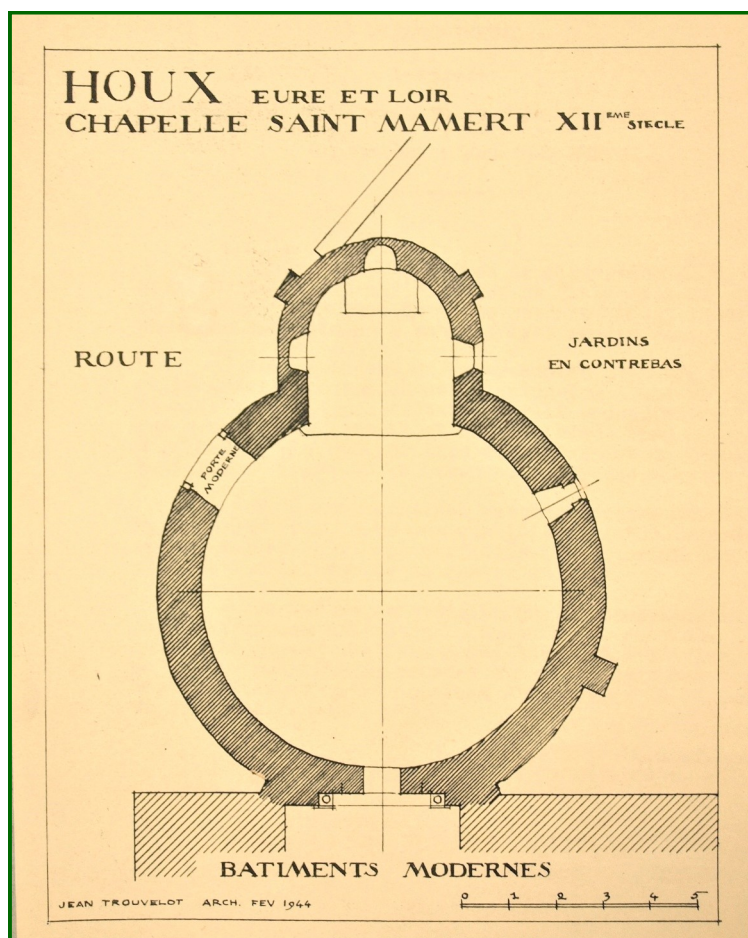
Plan de la chapelle en février 1944
