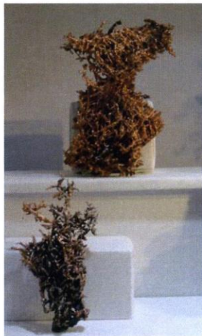
Gediegenes Kupfer
