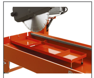
EFFIZIENTE SCHLAMMABSCHEIDUNG Die Schlammauffangschale ermöglicht eine effiziente Handhabung des Schlammes für eine lange Lebensdauer der Pumpe.
