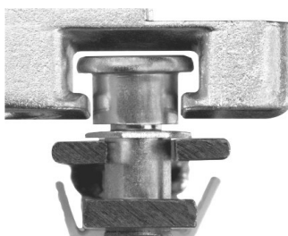
Pilzkopf-Verriegelung
