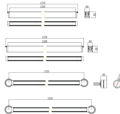
Medidas:(mm) 40W/50W
